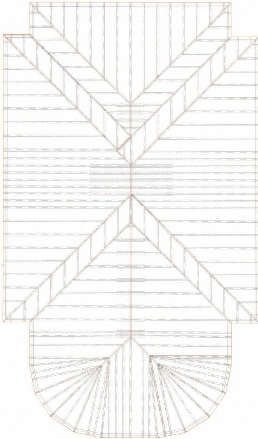
PLAN DE TOITURE
